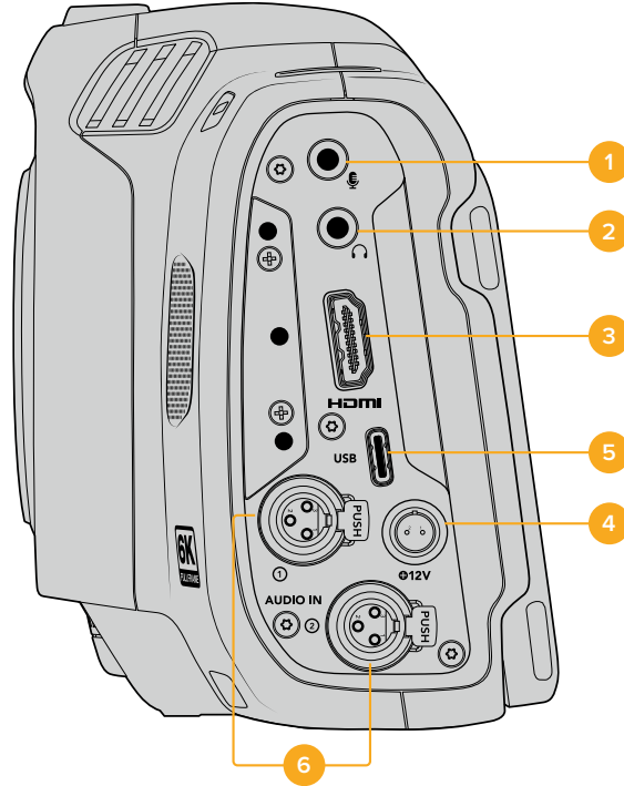
Blackmagic Cinema Camera 6K'nın sol tarafındaki portlar
