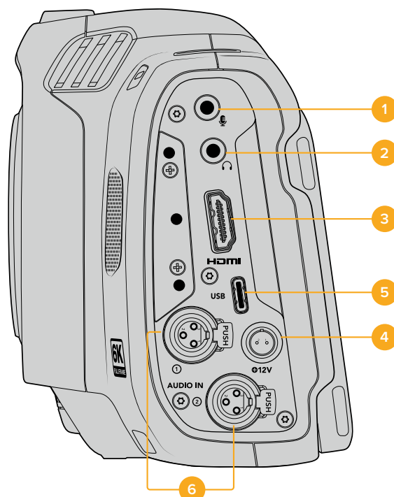
Порты на левой стороне модели Blackmagic Cinema Camera 6K
