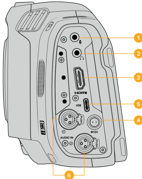
Blackmagic Cinema Camera 6K의 왼쪽 측면에 있는 단자 모습
