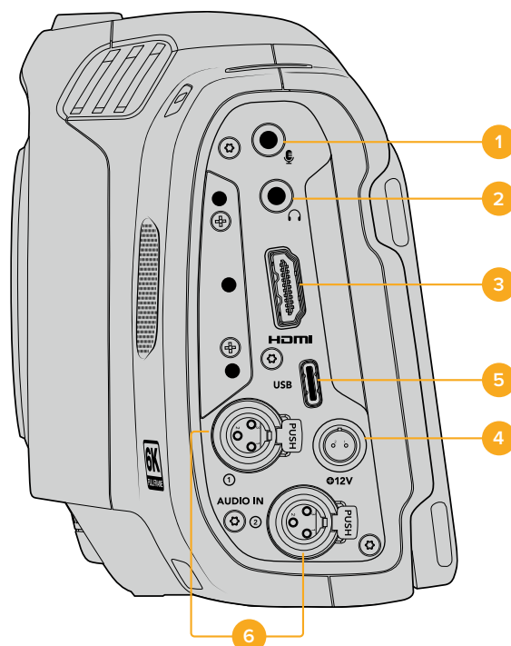
Puertos en el lateral izquierdo del modelo Blackmagic Cinema Camera 6K
