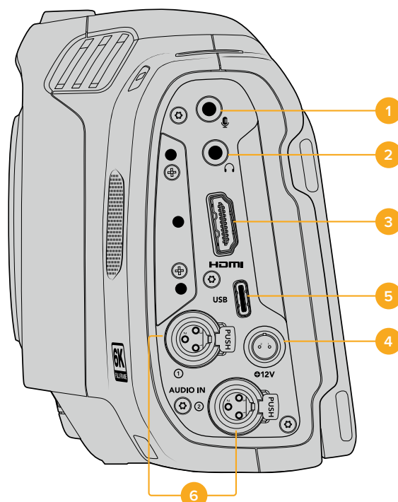
Blackmagic Cinema Camera 6K机身左侧端口示意图
