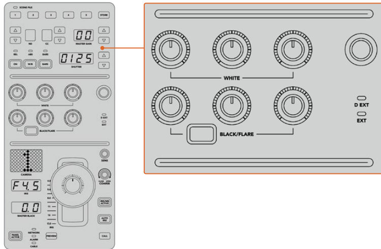
Die Farbabgleichregler dienen zur Feinjustage an den Rot-, Grün- und Blaukanälen für die Werte MASTER-Gain/Weiß, Gamma und Schwarzabhebung/Schwarzabhebung
