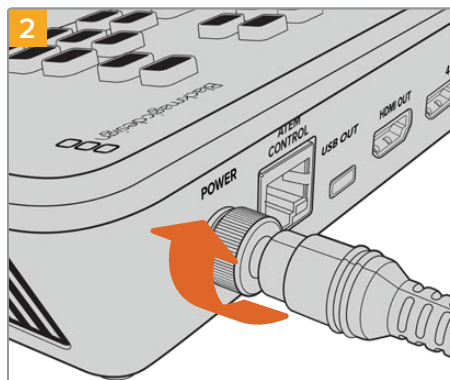
2 Закрутите разъем по направлению к ATEM Mini
