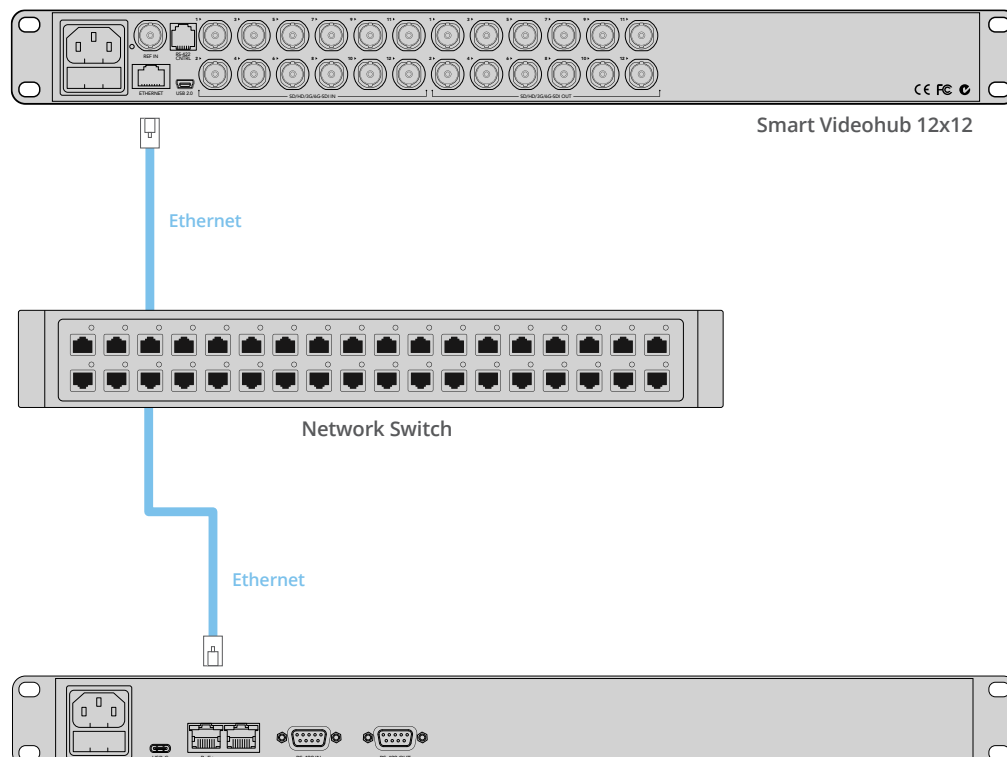
Ein per Ethernet-Switch an eine Smart Videohub 12x12 gekoppeltes Videohub Smart Control Pro Steuerpanel
