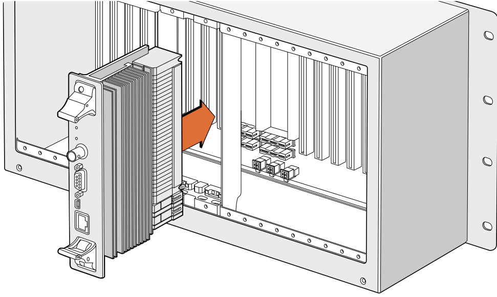
Universal Videohub 72 Crosspoint Cart'ın Takılması
