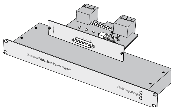
Il modulo Universal Videohub Power Supply di 1 RU include una scheda di alimentazione e un cavo
