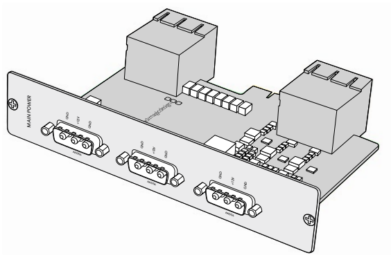
La scheda di alimentazione Universal Videohub da 450W ospita 3 connettori per alimentatori da 150W
