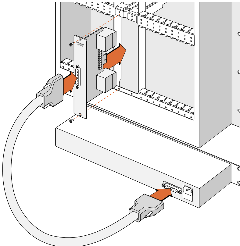
Universal Videohub Power Supply는 Universal Videohub 288에 삽입하는 1개의 카드와 이 카드를 연결해 Universal Videohub 288 하단에 장착하는 1RU 크기의 새시로 구성되어 있습니다.
