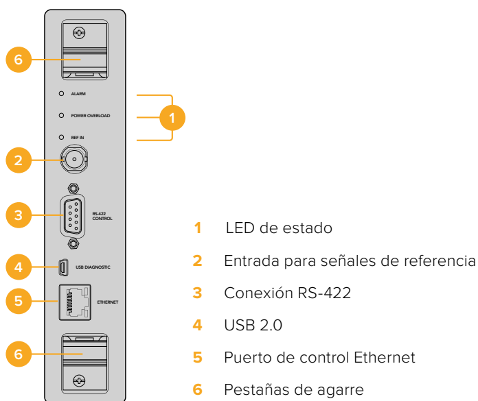
Tarjeta de puntos de cruce Universal Videohub 72 Crosspoint
