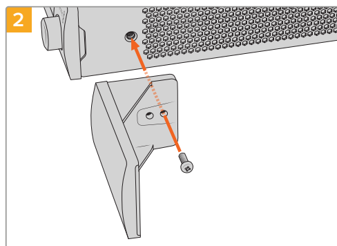
2 ブラックパネルをネジ穴に挿え、同梱のM3 (9mm) ネジで固定します。
