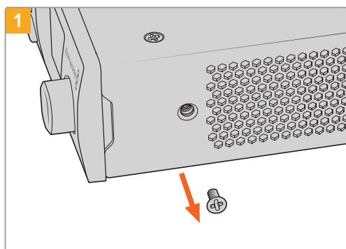
1 Wyręć śrubę M3 5 mm znajdującą się z przodu urządzenia
