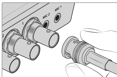
Подключите источники сигналов к SDI-входам микшера
