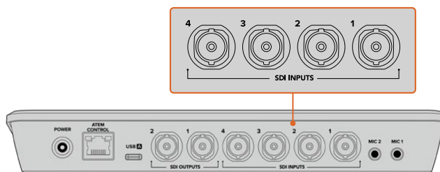
Schließen Sie SDI-Quellen an die SDI-Eingänge Ihres Mixers an
