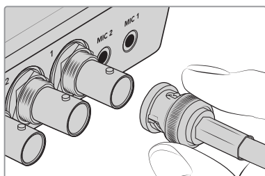
Schließen Sie SDI-Quellen an die SDI-Eingänge Ihres Mixers an
