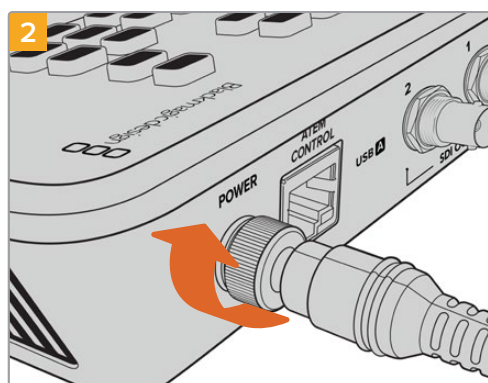
2 Avvita l'anello di bloccaggio per collegare il cavo saldamente
