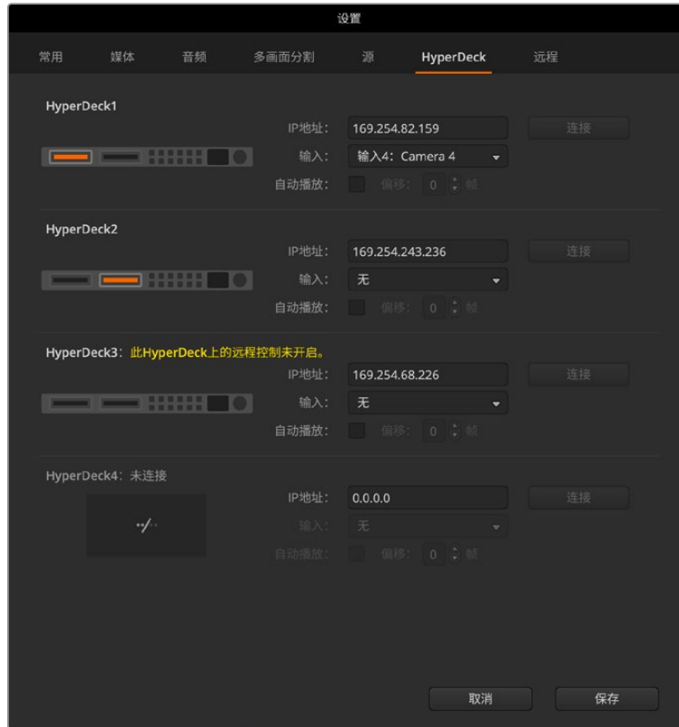
HyperDeck的各项设置
