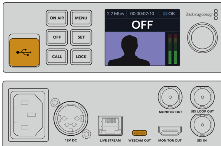
Blackmagic Web Presenter의 전면 또는 뒷면 패널에 있는 USB 포트를 사용하여 컴퓨터에 연결하세요.
