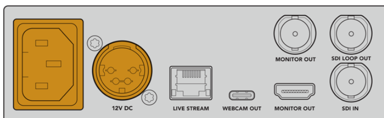
Blackmagic Web Presenterは、IECまたは12V DC電源入力から給電可能
